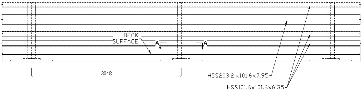
ELEVATION
